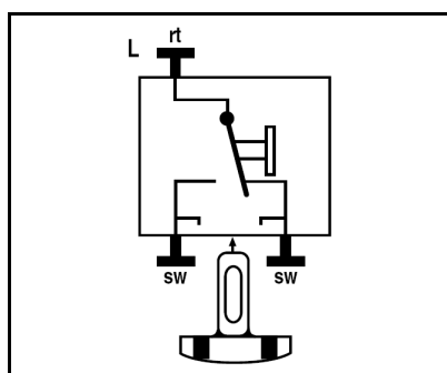
Contact aansluitingen
