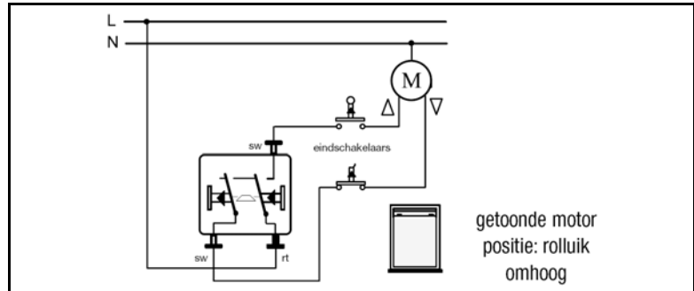
Schakelschema 809 VW
